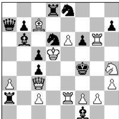
s # 2*v (12 + 13)
