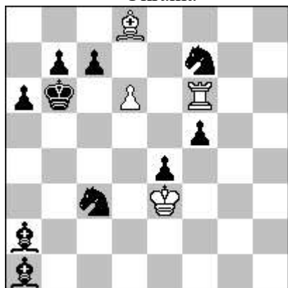
hs # 4,5 (4 + 10)
