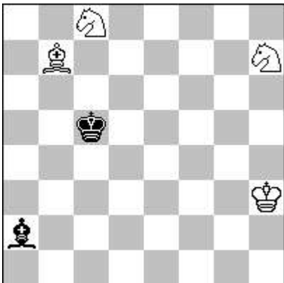
h # 4 3.1.1... (4 + 2)
