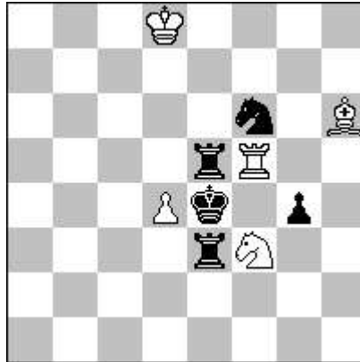
h # 2 3.1.1.1 (5 + 5)
