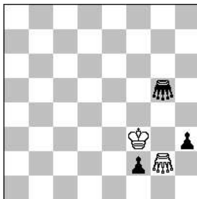
hs # 5 2.1.1... (2 + 3)
