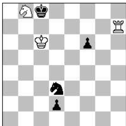
hs # 4 2.1.1... (3 + 4) Kōko
