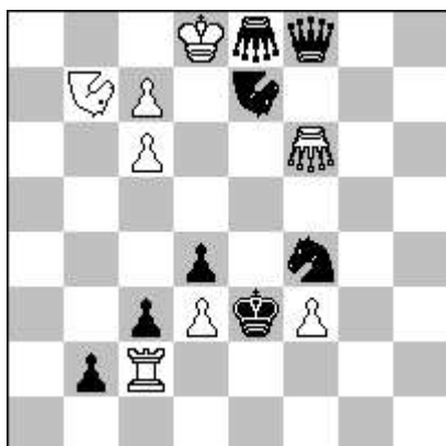
h # 2 2.1.1.1 (8 + 8) Madrasi
