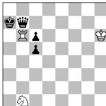
h # 2,5 0.2.1.1.1 (3 + 4) Circe
